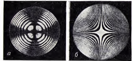
Рис. 5. Интерференционные картины хроматической поляризации в сходящихся лучах при условии, что оптические оси анализатора и поляризатора скрещены ( N_1 \perp N_2 , см. рис. 4). а — срез кристаллической пластинки K перпендикулярен её оптической оси; б — срез параллелен оптической оси. Если падающий на анализатор свет — белый, картины приобретают сложную характерную окраску.
